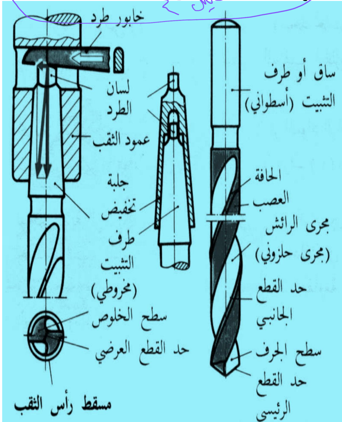
شكل (24-3) أجزاء البريمة الحلزونية
