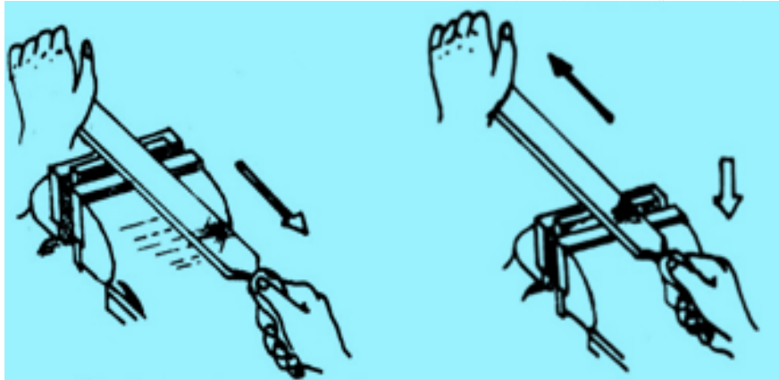
الشكل (2-3) عملية القطع بالمبرد
