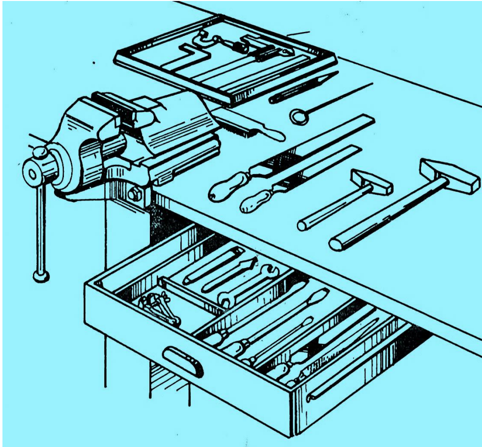
شكل (7-3) منضدة البرادة وتنظيم أدوات البرادة
