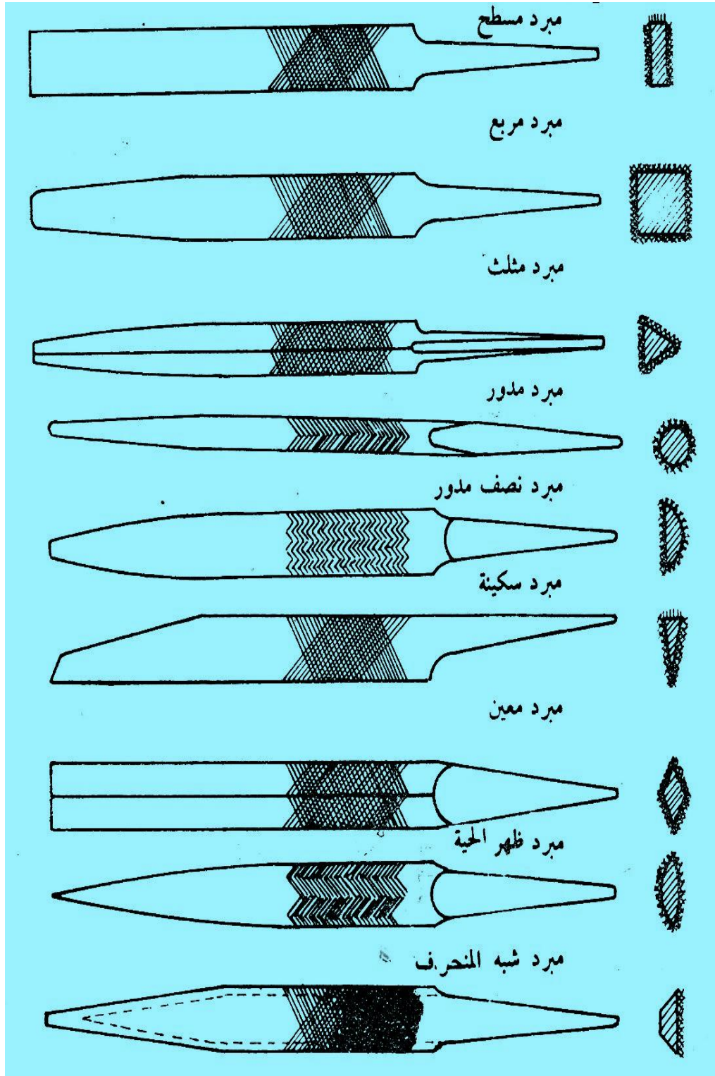
شكل (3-6) أشكال مقاطع المبرد
